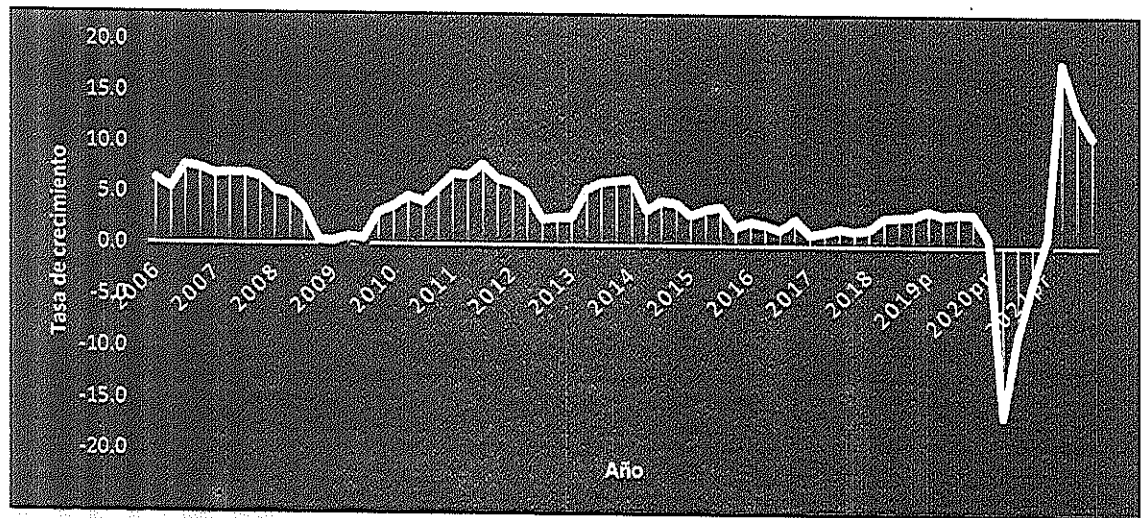
FUENTE. (DANE, 2022)
